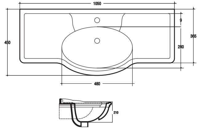
40127 Lavabo cm 70 Washbasin cm 70 Lavabo cm 70
